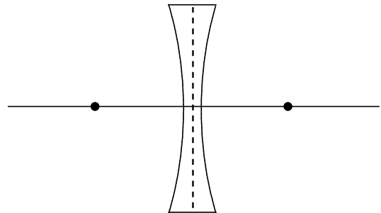
凹レンズ
