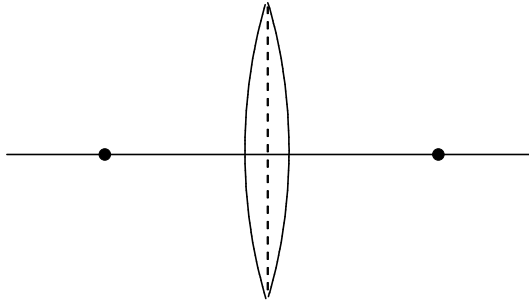
凸レンズ
